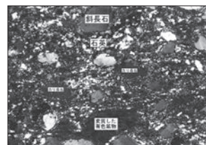
写真7 No.168 マイロナイト鏡下写真 (偏光板2枚挿入)
