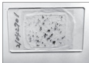
写真2 岩石薄片
