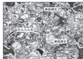
写真4 No.60 かんらん岩鏡下写真 (偏光板1枚挿入)
