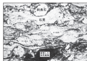
写真6 No.168 マイロナイト鏡下写真 (偏光板1枚挿入)
