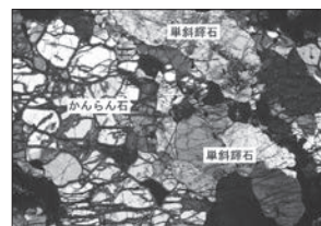
写真5 No.60 かんらん岩鏡下写真 (偏光板2枚挿入)
