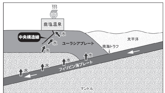
図2 鹿塩温泉の水が地上に湧き出るまでの経路
