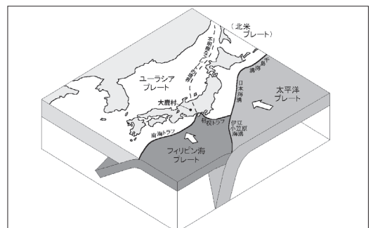
図1 日本周辺のプレートの位置 防災科学技術研究所ホームページに加筆 原図は、萩原尊禮編「日本列島の地震、地震工学と地震地体構造」鹿島出版会
