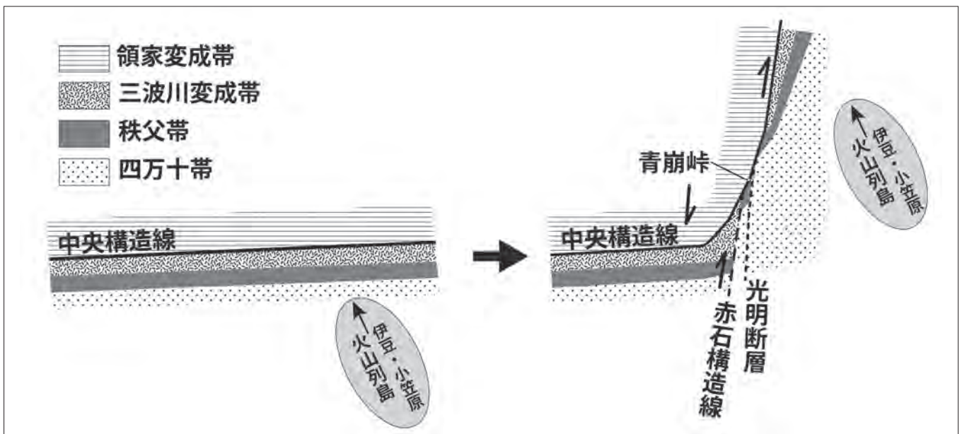
図2 1500万年前頃、伊豆・小笠原火山列島の衝突により、南アルプス地域の中央構造線は曲がり、新しくできた赤石構造線、光明断層と共に60kmに渡って左横ずれしたイメージ図
